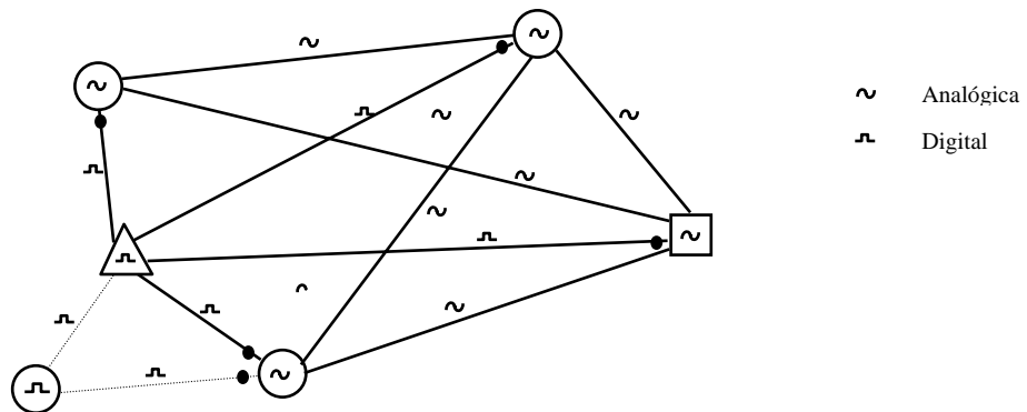
Figura 16: Extensión con nueva central local
