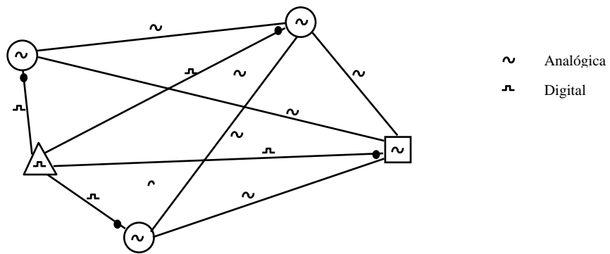
Figura 15: Tándem analógico desfasado
