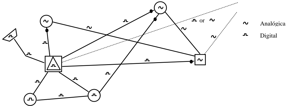
Figura 23: Introducción de funciones de tránsito en una central tándem digital existente
